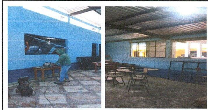
Foto 5: Sustitucion de ventanas de estructura de metal con vidrio de 5mm de 2.00 mts x 1.10 mts
